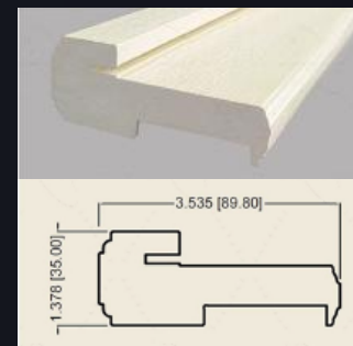
OTG005- Astragal
