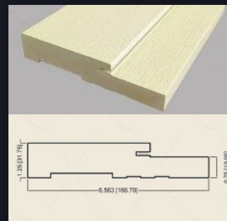
OTG003- 6-9/16" Jamb
